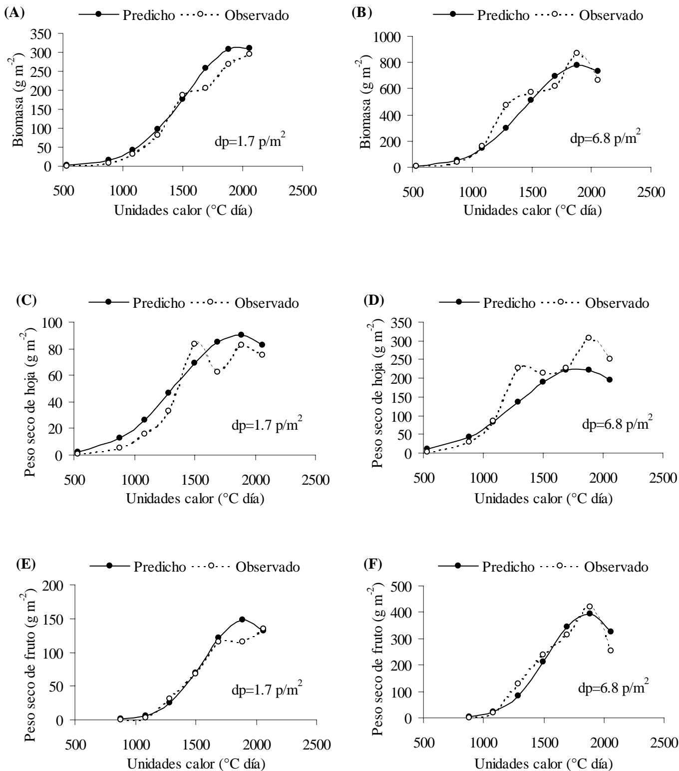
Figura 2. Cinética de crecimiento en biomasa total, peso seco de hoja y peso seco de fruto en las densidades de 1.7 y 6.8 plantas/ m^2 , con datos observados y predichos con la modificación a la función de Gauss. Se indica como dp = densidad de plantas/ m^2 .
